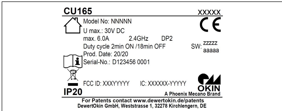
Abbildung 1 Typenschild CU165 (Beispiel)
