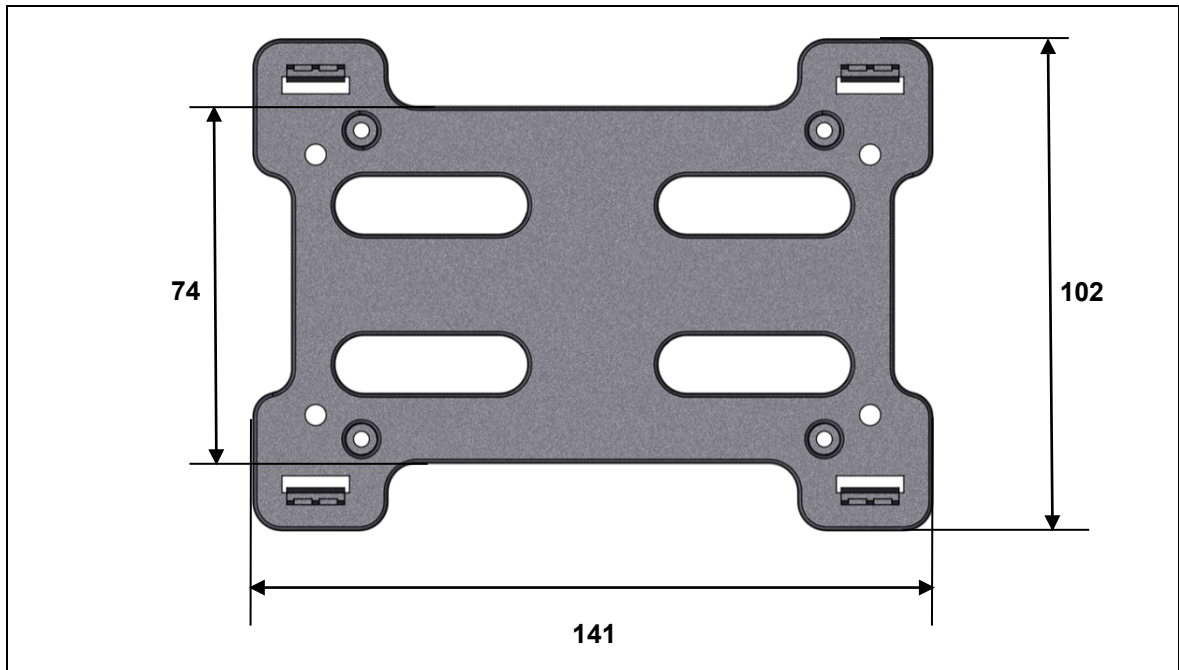
Abbildung 5 Maße der Montageplatte, Draufsicht (Angaben in mm)
