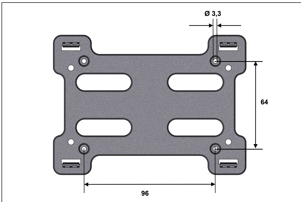
Abbildung 7 Bohrmaße (Beispiel): Befestigungspunkte an der Montageplatte (Angaben in mm)
