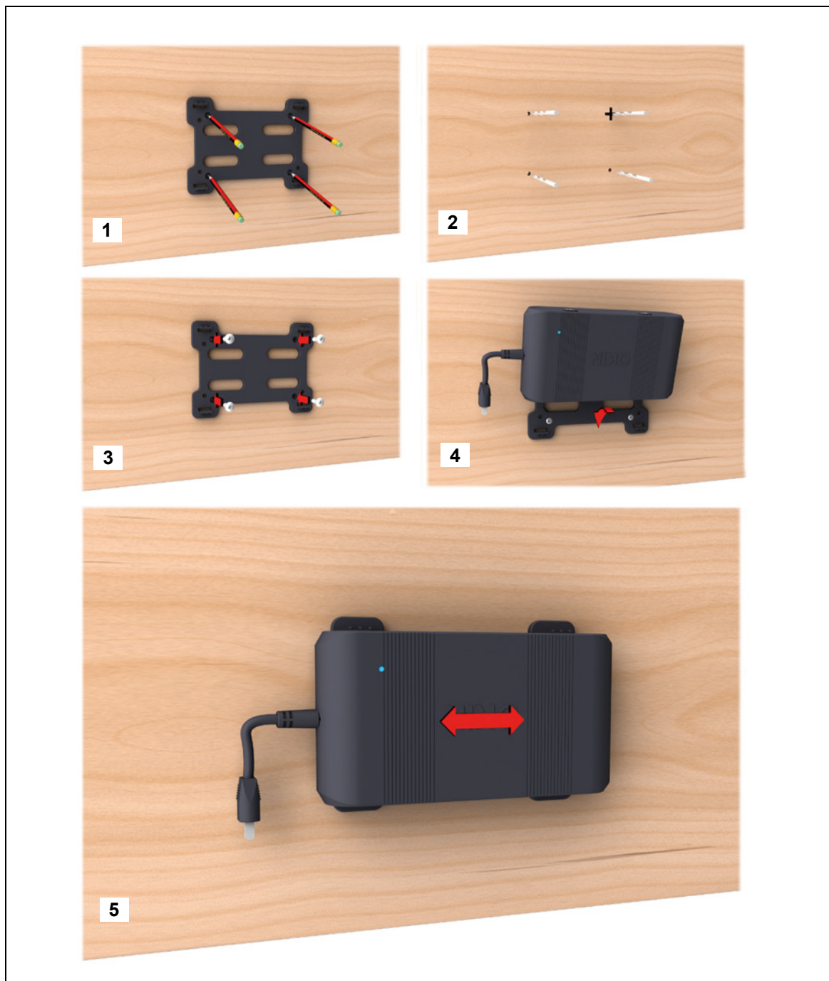
Abbildung 8 Montage der der Montageplatte und Befestigung der CU165
