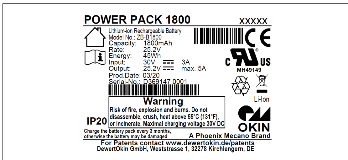
Abb. 2: Typenschild POWER PACK 1800 (Beispiel)
