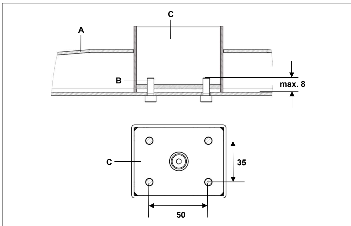
Abbildung 8 Montage Tischfuß (Variante A): (Angaben in mm)
