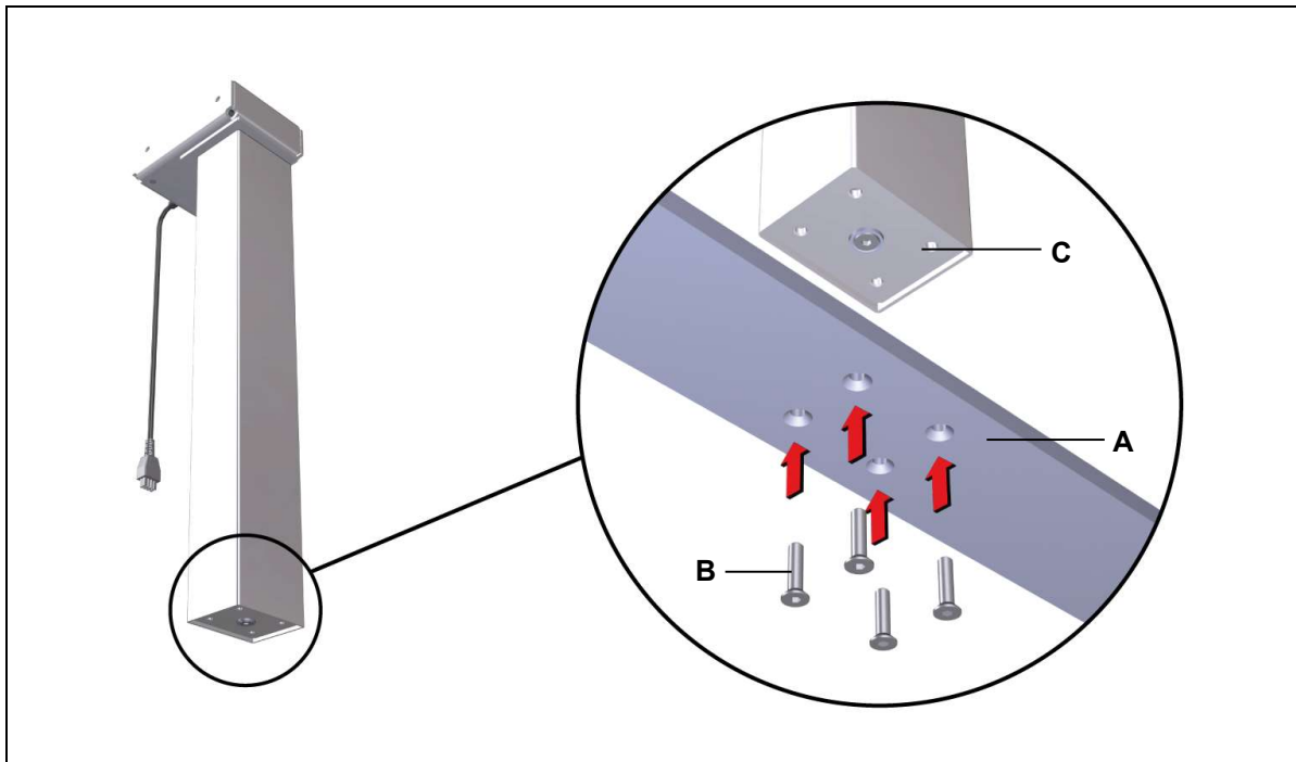
Abbildung 13 Beispiel: Montage Tischfuß (Variante D)
