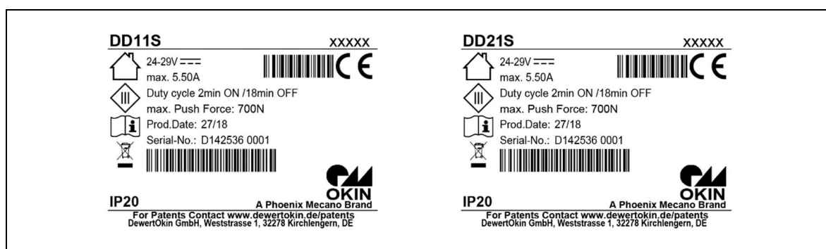
Abbildung 2 Typenschilder (Beispiele)
