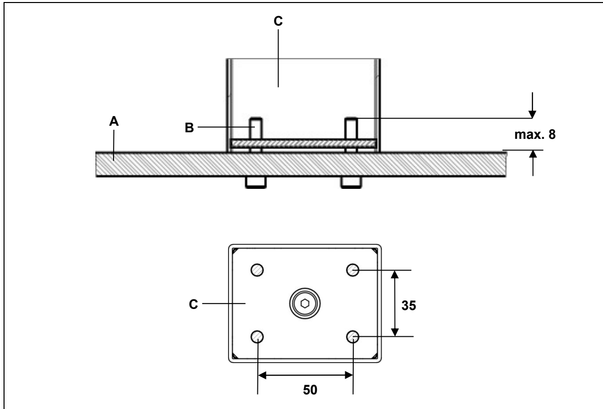
► Abbildung 10 Montage Tischfuß (Variante B) (Angaben in mm)
