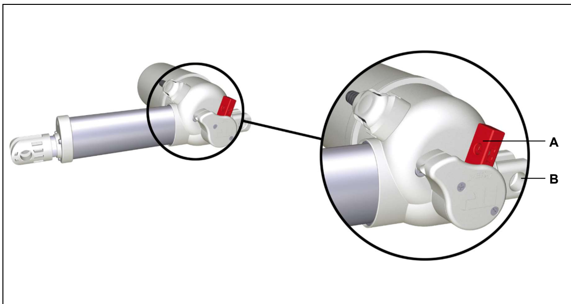
Abbildung 10 Antrieb MEGAMAT MCZ mit Rückstellfunktion (ER) mit Bowdenzuganbindung
