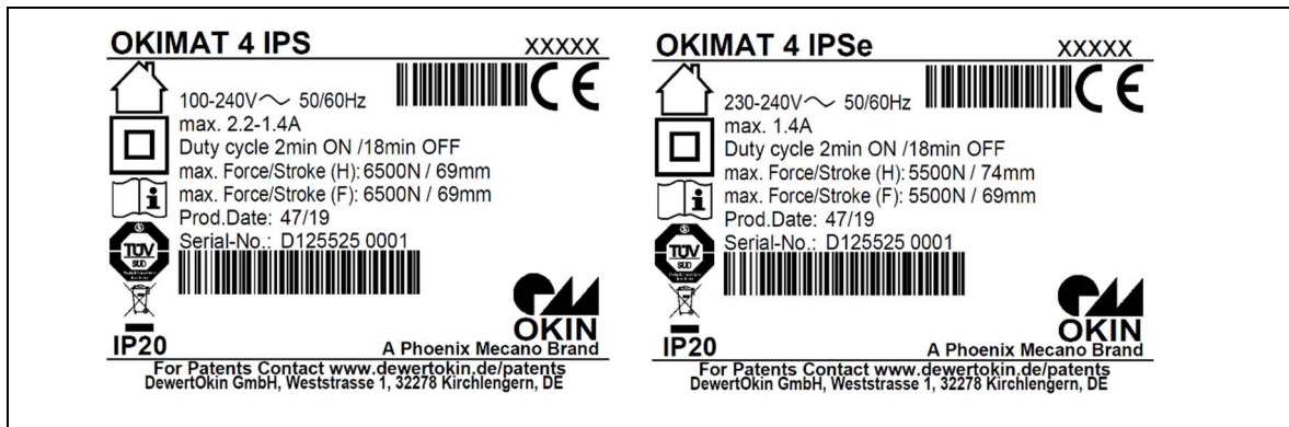
Abbildung 2 Typenschilder (Beispiele)
