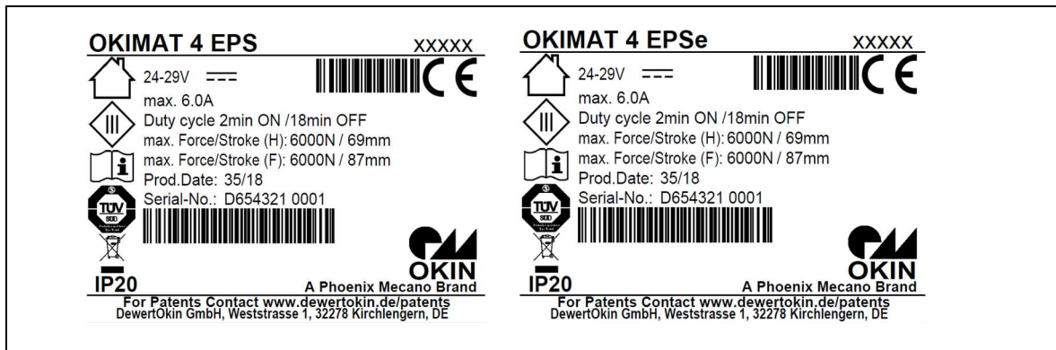
Abbildung 3 Typenschilder (Beispiele)
