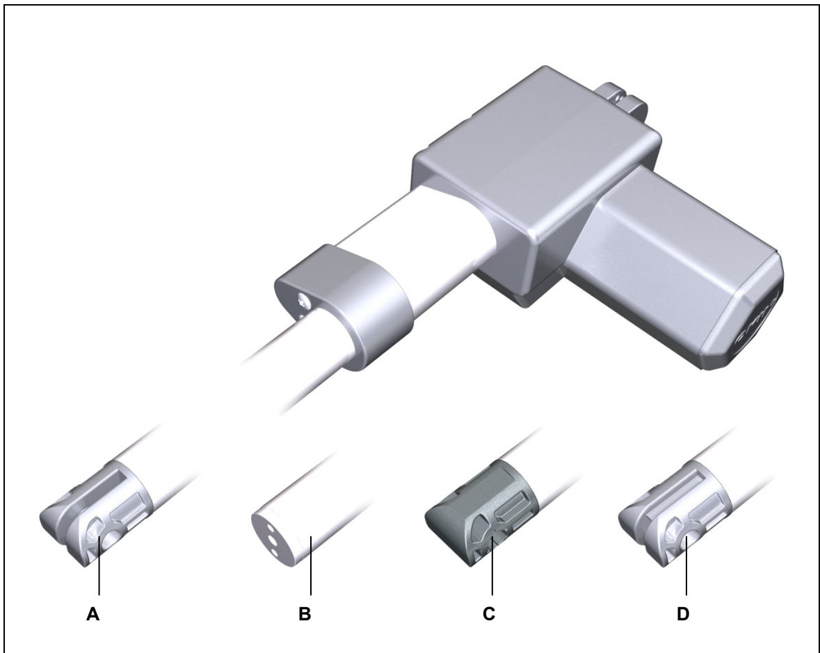
Abbildung 3 Gabelkopf-Varianten
