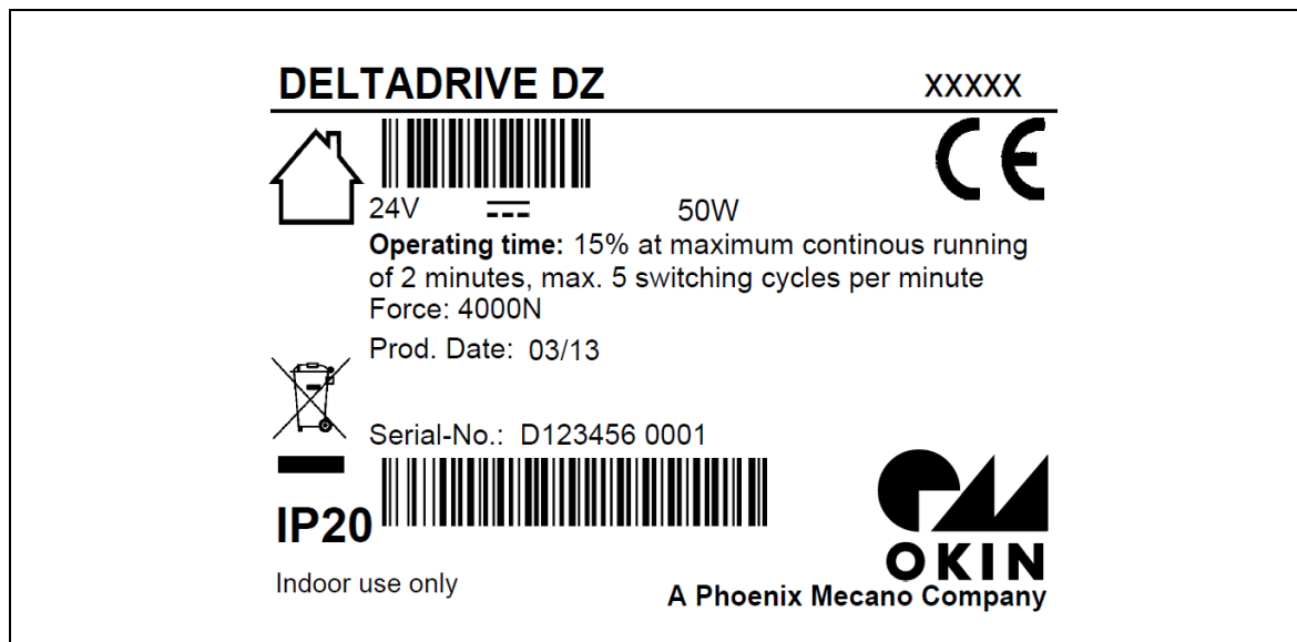
Abbildung 1 Typenschild (Beispiel)
