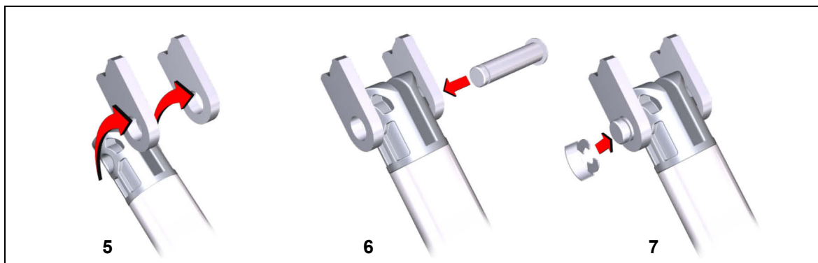
Abbildung 14 Montageschritte am Hubrohrkopf (Beispiel)
