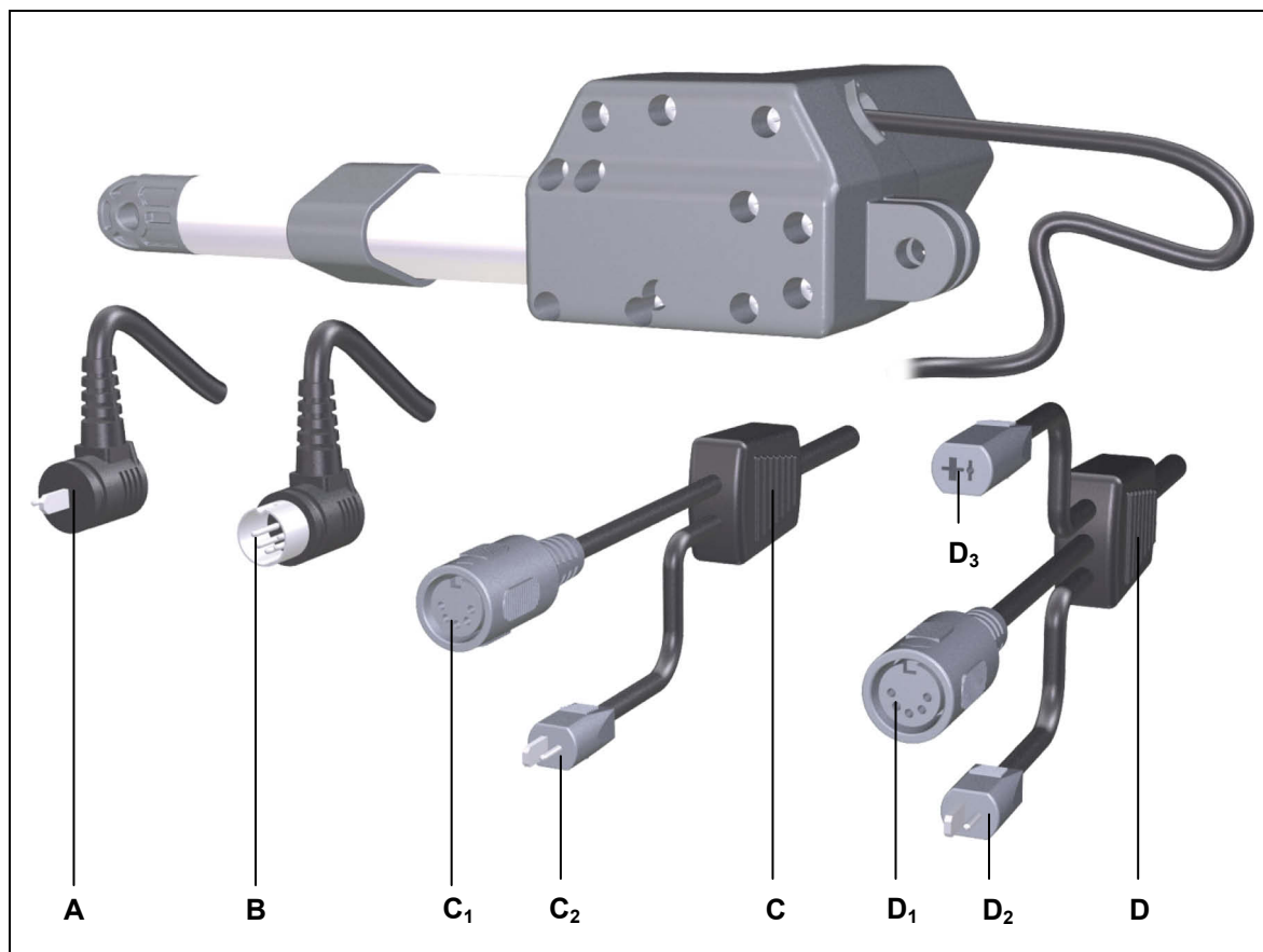
Abbildung 7 Varianten der Stecker und Kabel für verschiedene Antriebstypen DELTADRIVE
