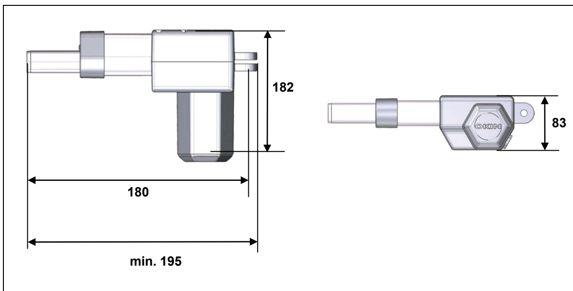
Abbildung 9 Maße des Antriebs DELTADRIVE mit Adapter (Angaben in mm) Mindest-Einbaumaß: 180 mm
