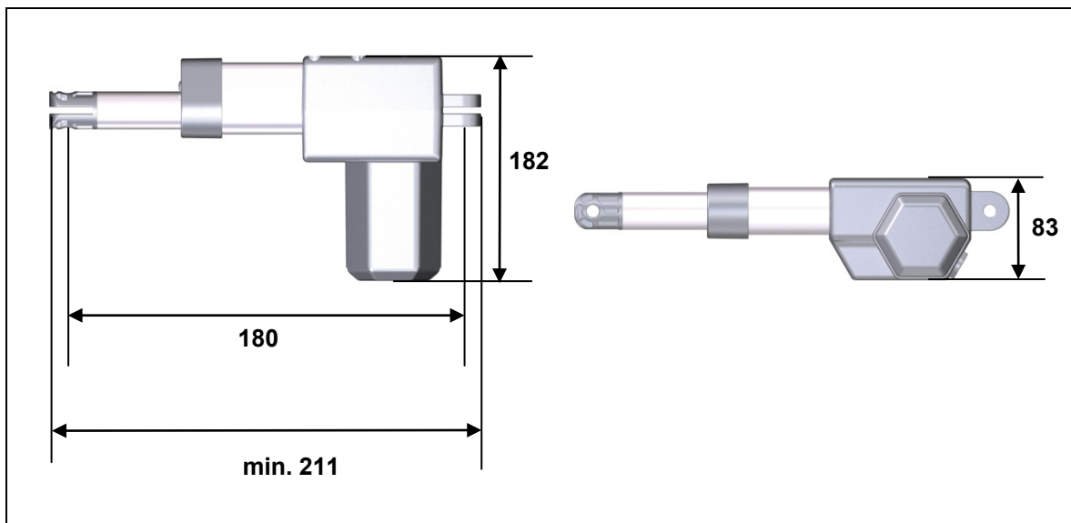
Abbildung 8 Maße des Antriebs DELTADRIVE mit Hubrohgabelkopf (Angaben in mm) Mindest-Einbaumaß: 180 mm
