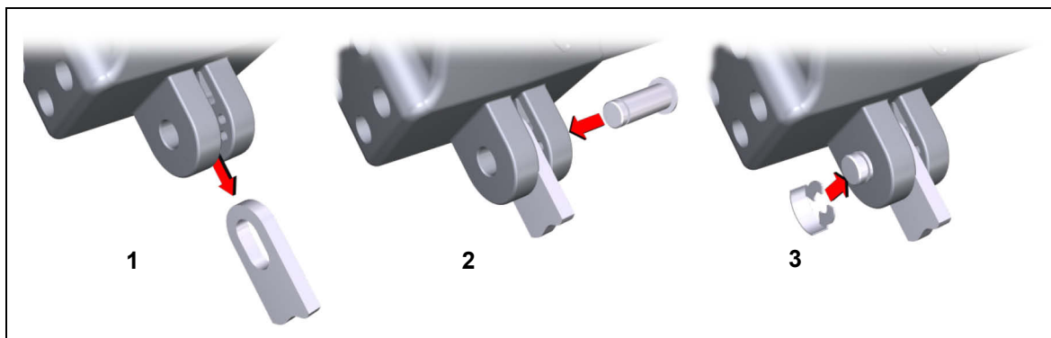
Abbildung 13 Montageschritte am Getriebegabelkopf (Beispiel)
