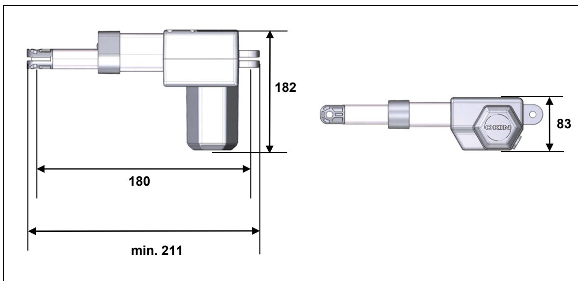
Abbildung 11 Maße des Antriebs DELTADRIVE mit Hubrohrkopf, Ausführung verstärkt (Angaben in mm), Mindest-Einbaumaß: 180 mm
