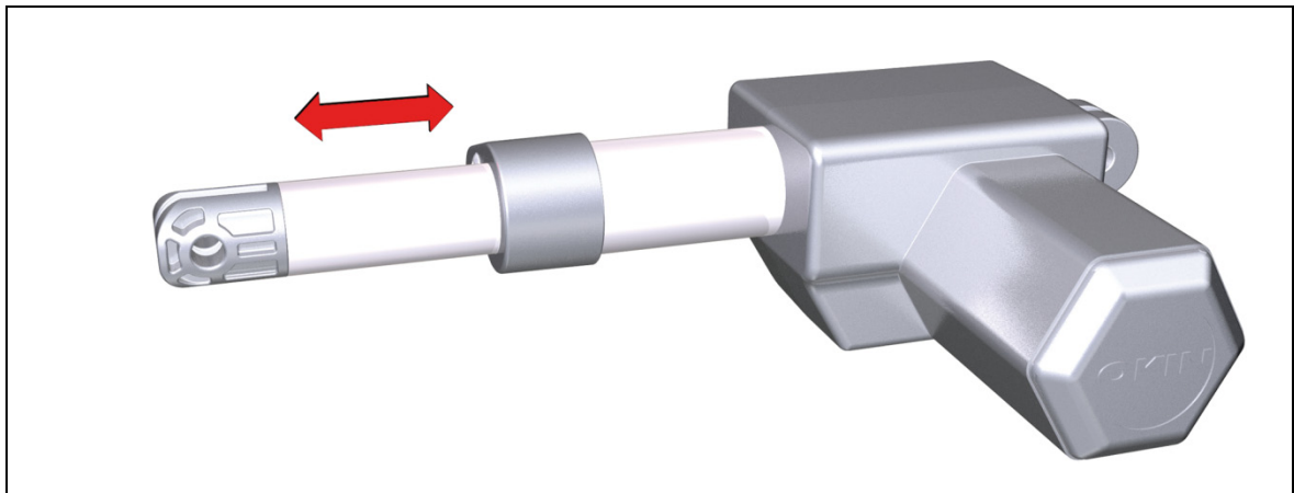
Abbildung 6 Fester Muttersitz = Hubrohr fest mit der Spindel verschraubt: Druck- und Zugkräfte
