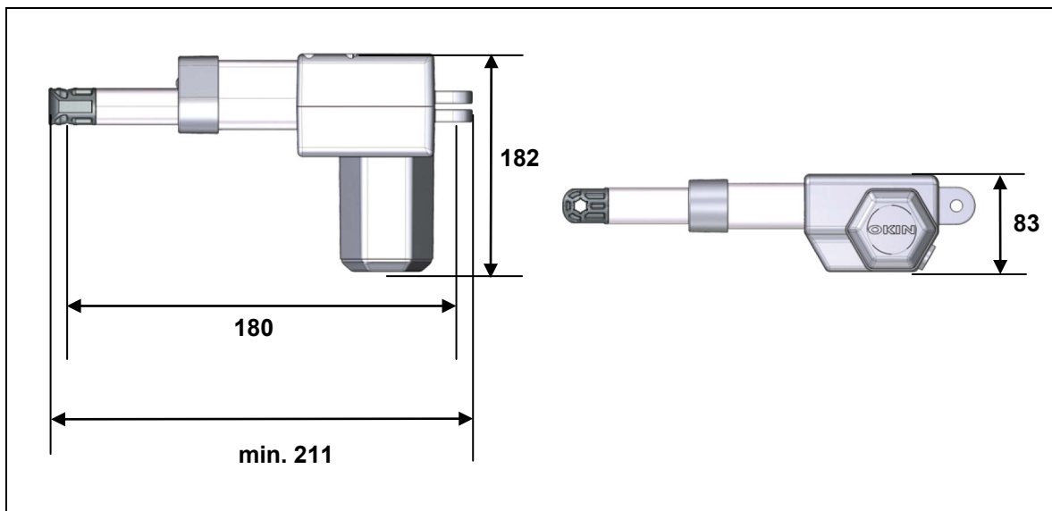
Abbildung 10 Maße des Antriebs DELTADRIVE mit Hubrohrkopf, Ausführung Guss (Angaben in mm), Mindest-Einbaumaß: 180 mm
