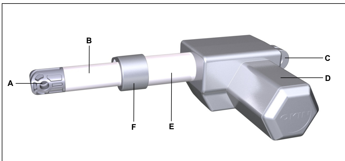
Abbildung 2 Hauptbestandteile des Antriebs DELTADRIVE
