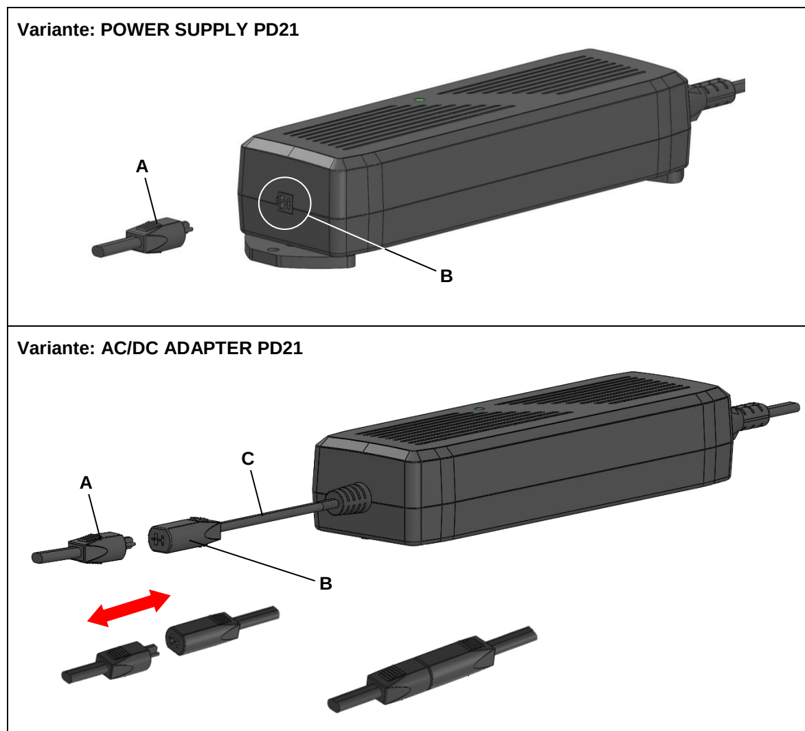
Abbildung 11 Anschluss für Antrieb/Antriebssteuerung
