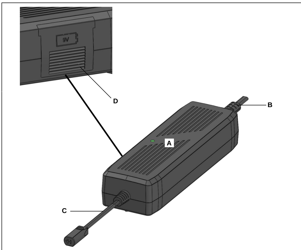
Abbildung 4 Komponenten des AC/DC ADAPTER PD21
