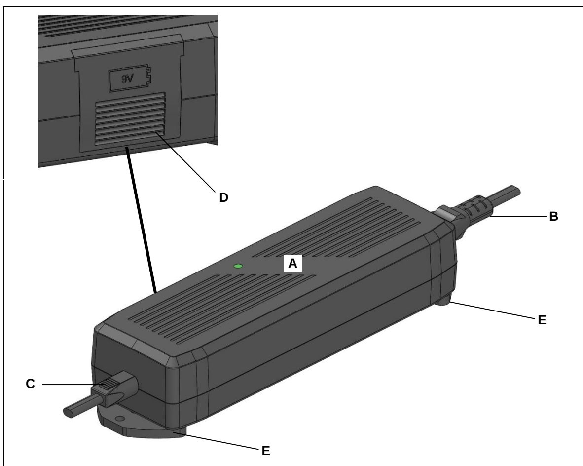
Abbildung 3 Komponenten des POWER SUPPLY PD21
