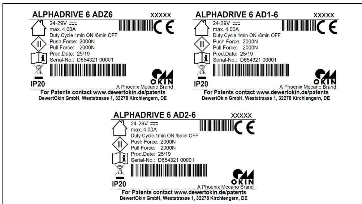
Abbildung 2 Typenschilder (Beispiele)
