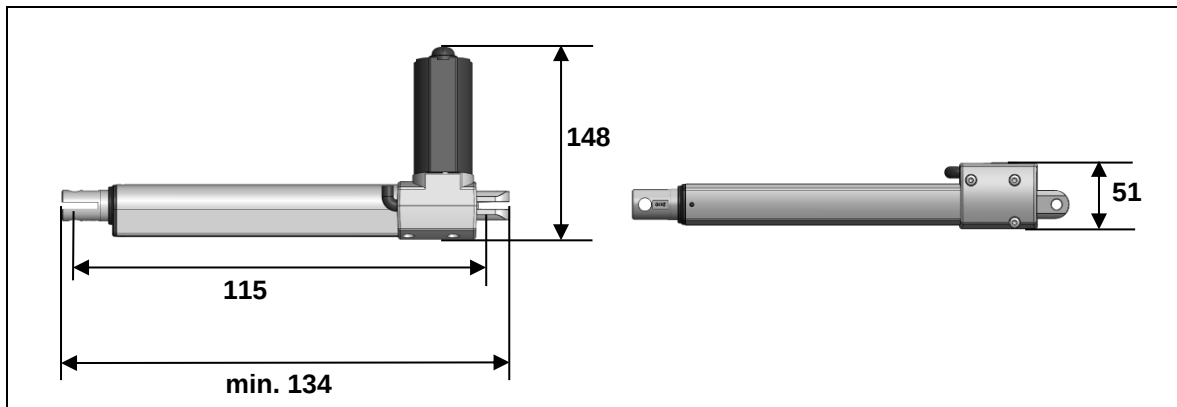
Abbildung 13 Maße des Antriebs MICRODRIVE 3 Hubrohgabelkopf (Metall) mit Schlitz (Angaben in mm) Mindest-Einbaumaß: 115 mm
