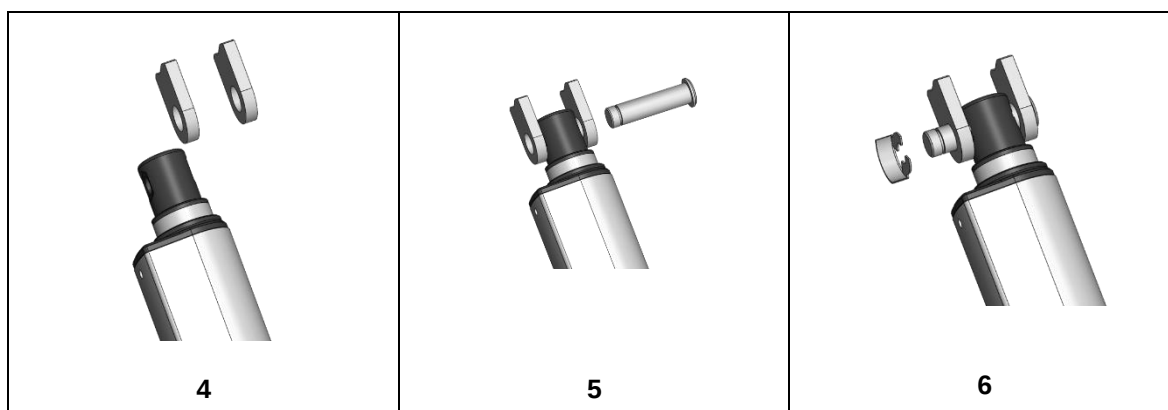
Abbildung 16 Montageschritte am Hubrohrkopf (Beispiel)
