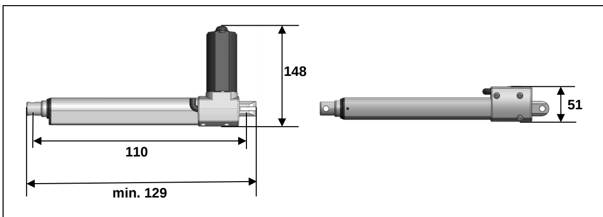
Abbildung 9 Maße des Antriebs MICRODRIVE 3 Hubrohrkopf (Metall) ohne Schlitz (Angaben in mm) Mindest-Einbaumaß: 110 mm
