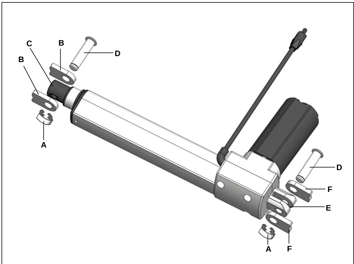
Abbildung 14 Einbau des Antriebs (Beispiel)
