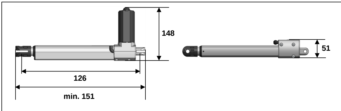
Abbildung 7 Maße des Antriebs MICRODRIVE 3 Hubrohgabelkopf (Schlitz 5mm) Mindest-Einbaumaß: 126 mm
