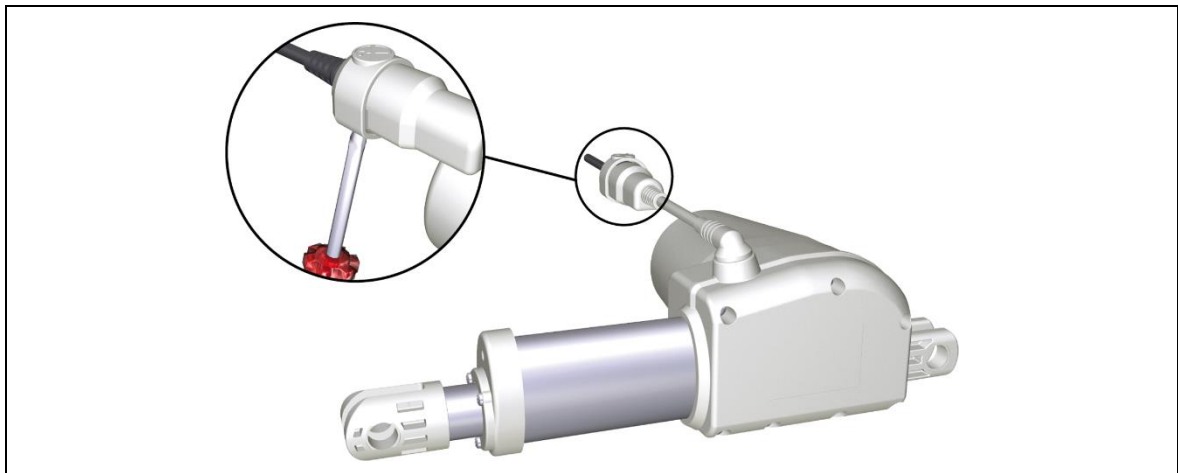
Abbildung 21 Lösbare Verriegelungskappe am Kabel in kurzer Ausführung
