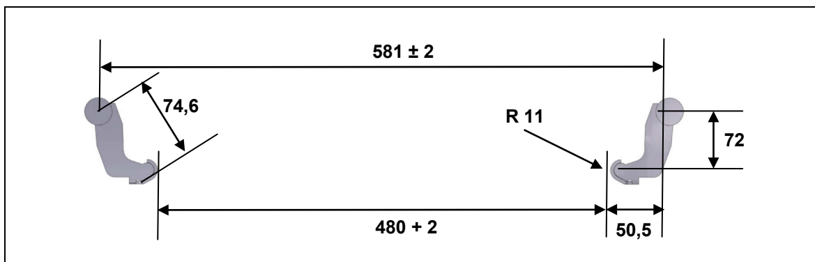
Abbildung 8 Lage Anlenkhebel (Angaben in mm)
