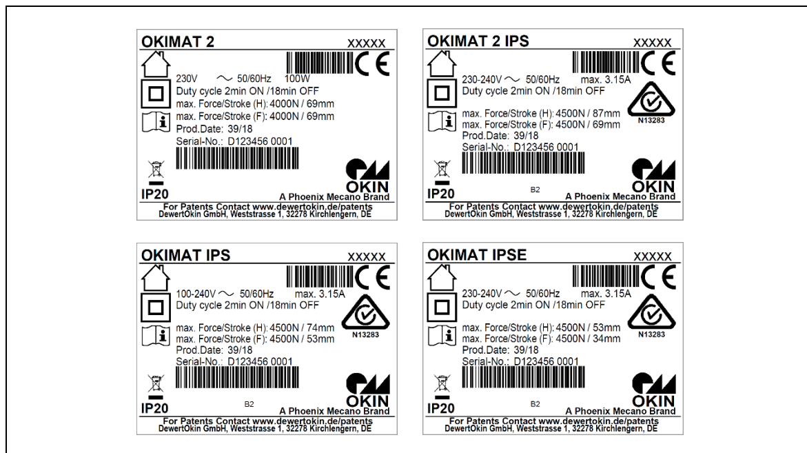
Abbildung 1 Typenschilder (Beispiele)
