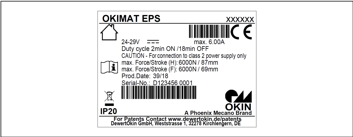
Abbildung 2 Typenschild (Beispiel)
