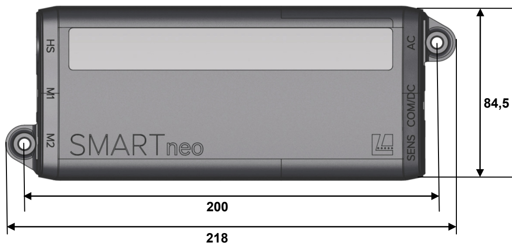
Abbildung 59 Steuerung SMARTneo / SMARTneo-pro, Draufsicht (Angaben in mm)
