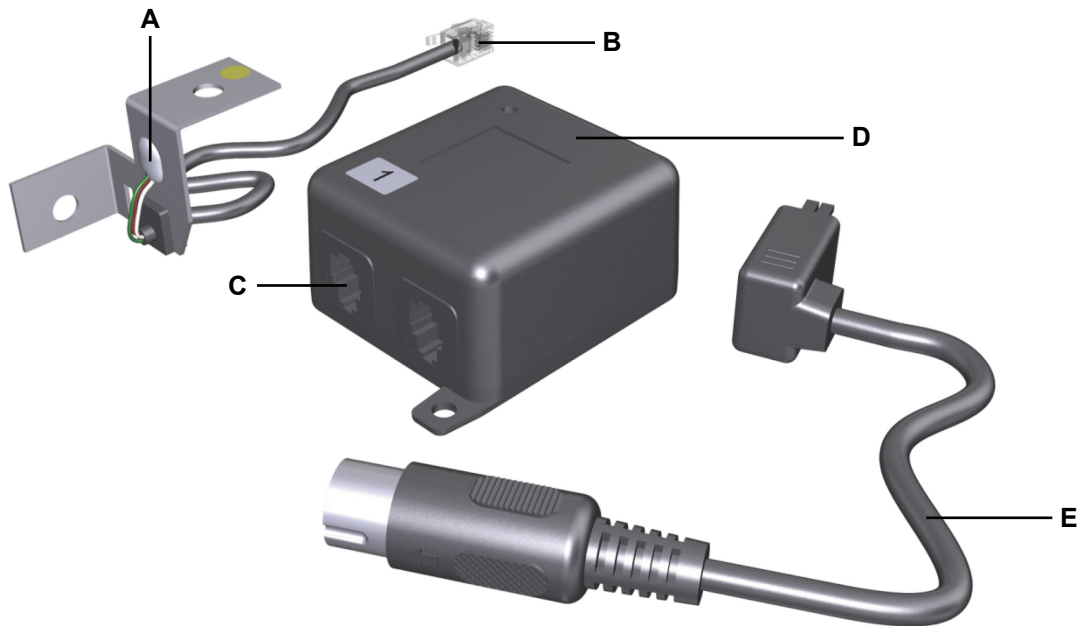
Abbildung 43 Sensoreinheit
