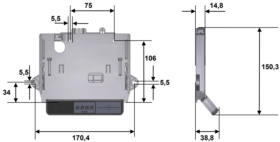
Abbildung 30 Bedienelement TOUCHdown, Montagemaße (Angaben in mm)
