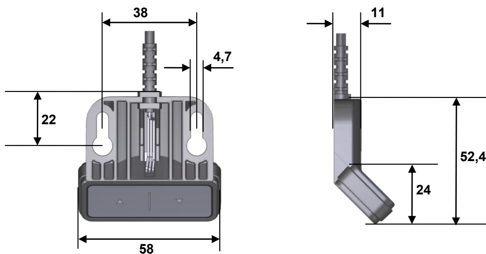
Abbildung 28 Bedienelement TOUCHbasic-down, Montagemaße (Angaben in mm)
