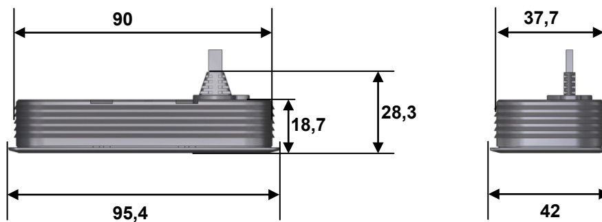
Abbildung 31 Bedienelement TOUCHinlay, Montagemaße (Angaben in mm)
