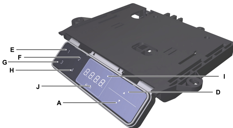
Abbildung 55 Bedienelement TOUCHdown
