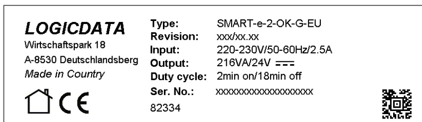
Abbildung 67 Typenschild (Beispiel)
