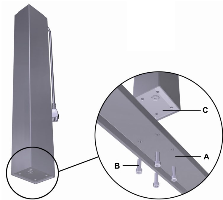
Abbildung 18 Montage Tischfuß
