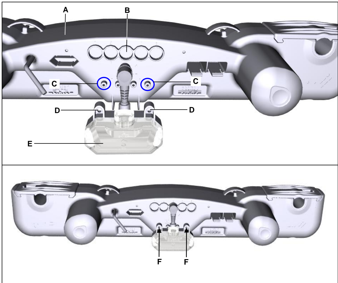
Abbildung 6 Montage am Doppelantrieb (Beispiel DUOMAT 8)
