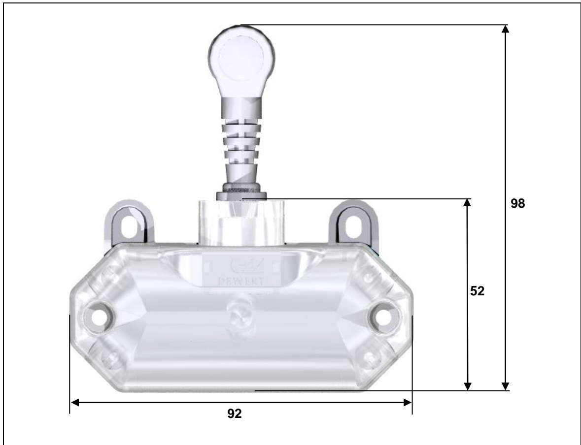
Abbildung 4 Maße der Unterbettbeleuchtung zum Aufstecken auf den Doppelantrieb (Angaben in mm)
