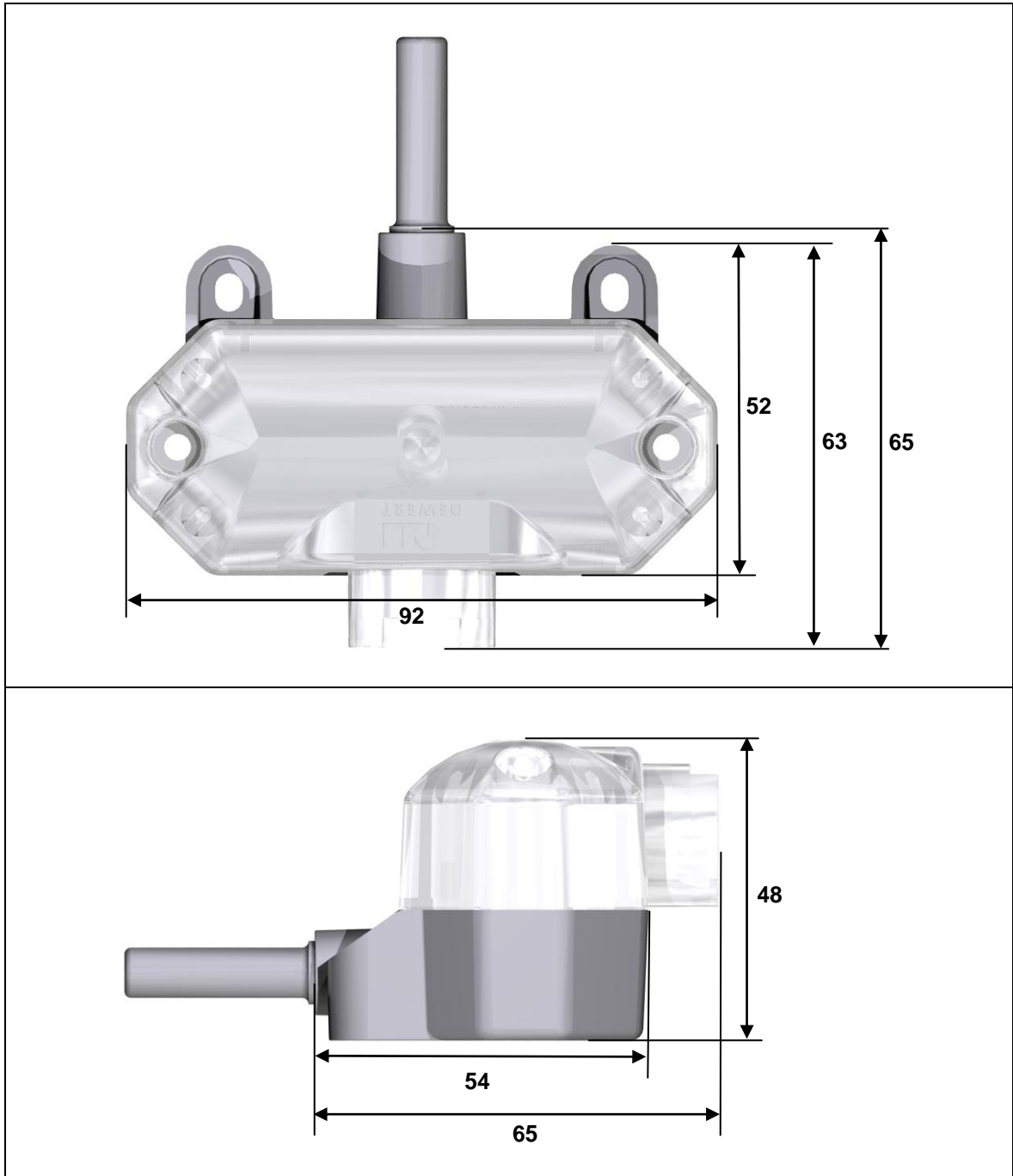
Abbildung 3 Maße der Unterbettbeleuchtung mit Handschalter-Buchse (Angaben in mm) und Kabelanschluss
