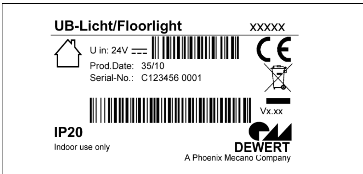
Abbildung 1 Typenschild (Beispiel)
