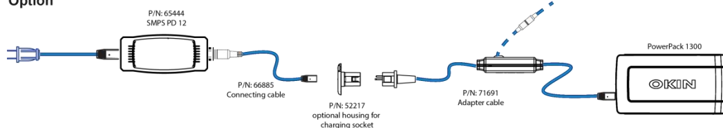
Abb. 06: Übersicht Lademöglichkeiten des POWER PACK 1300
