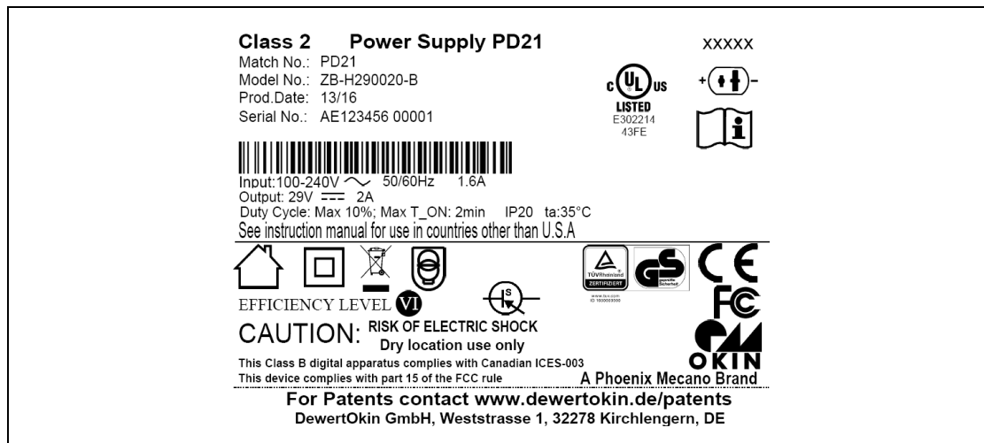
Abb. 1: Typenschild Power Supply PD21 (Beispiel)
